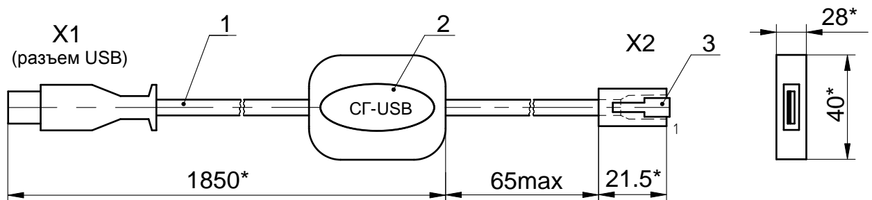
Рисунок Г.3 – Соединение гибкое СГ2
