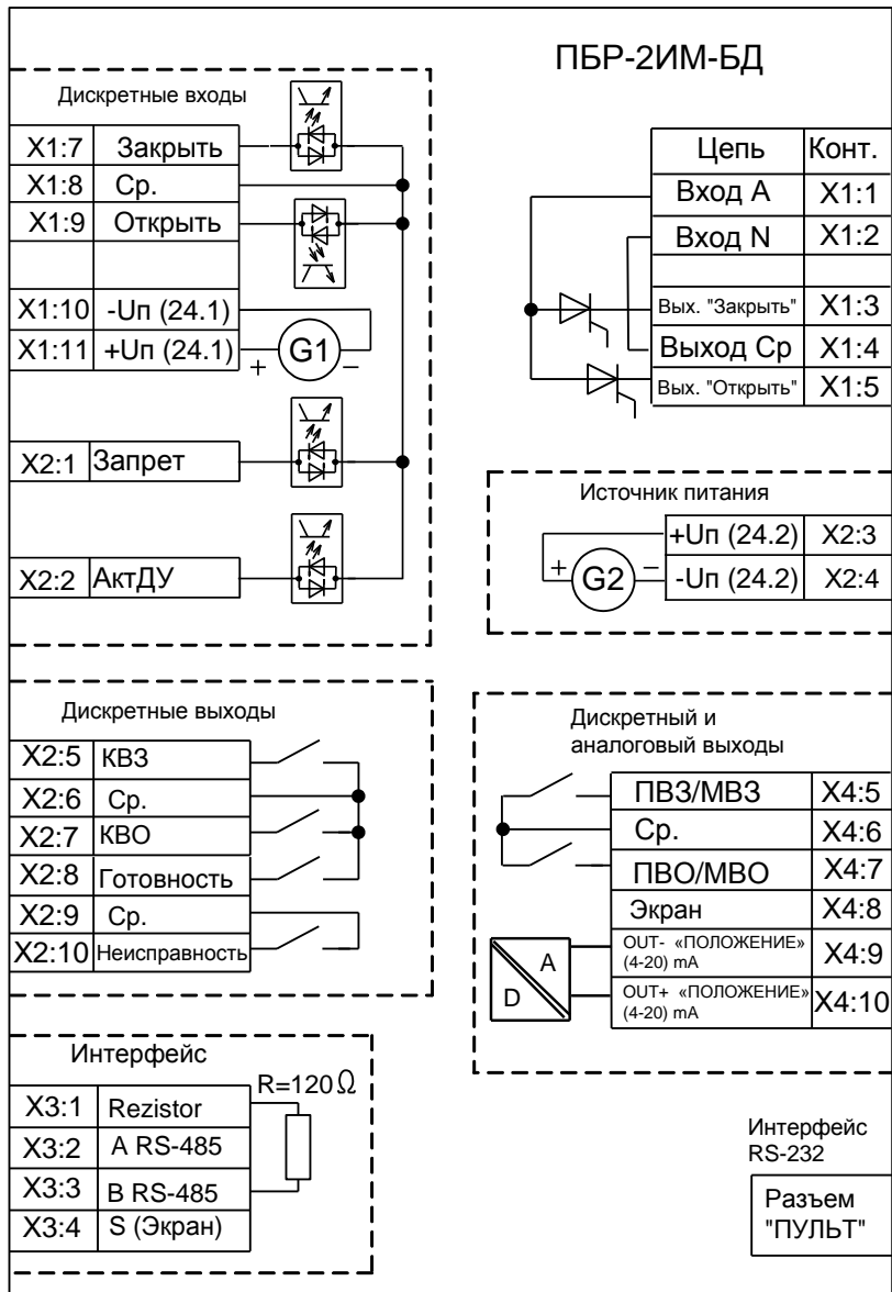
Рисунок Н.3 – Схема ПБР-2ИМ-БД-XX-ДУ
