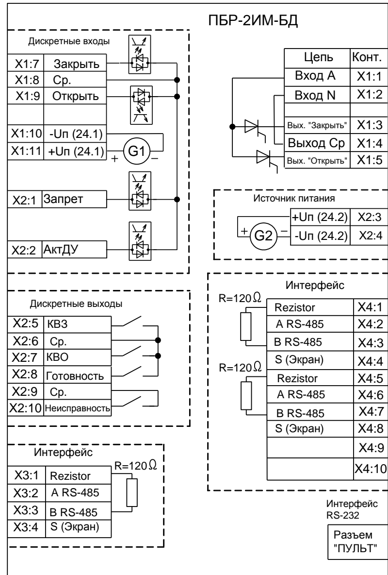
Рисунок Н.8 – Схема ПБР-2ИМ-БД-ХХ-2С
