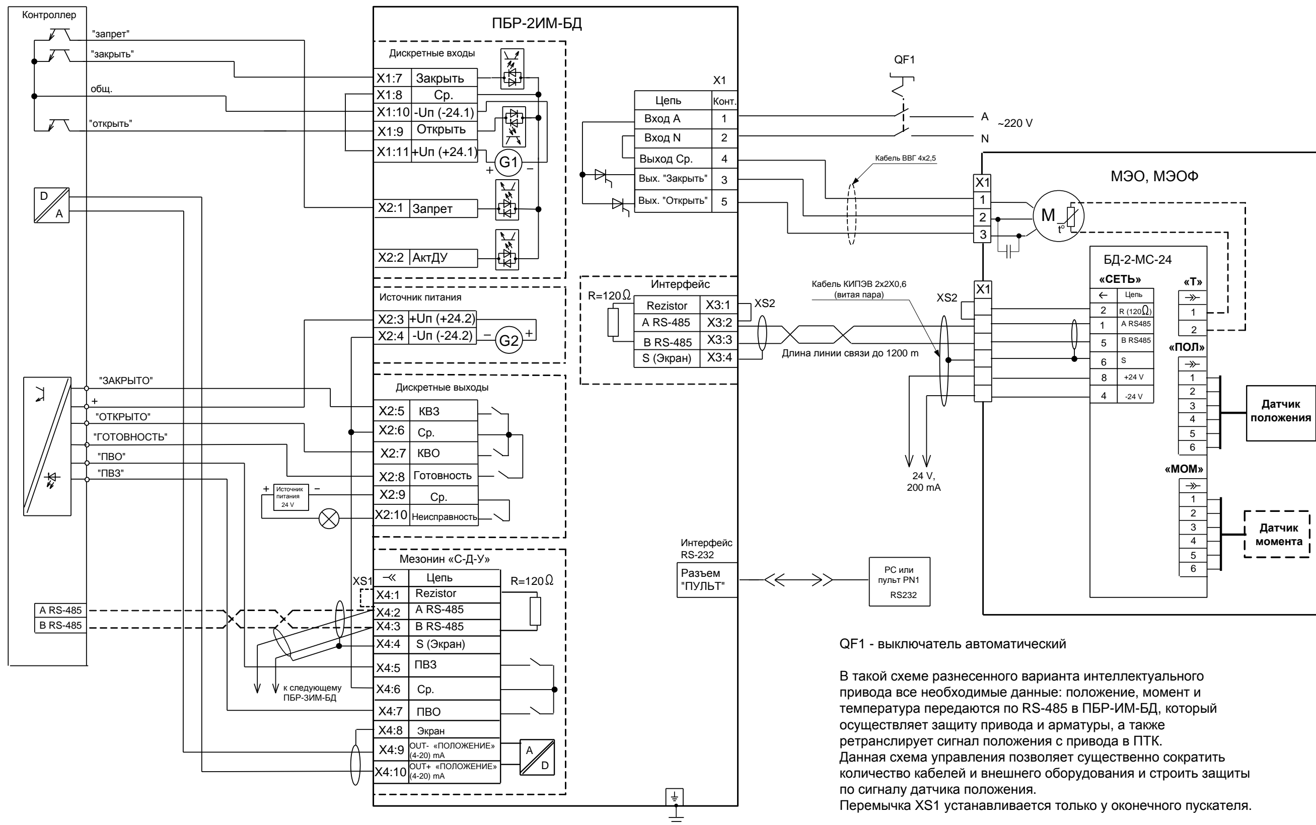
Рисунок П.2 – Схема управления ЭП с использованием пускателя ПБР-2ИМ-БД-ХХ-СДУ и блока датчиков БД-2-МС-24
