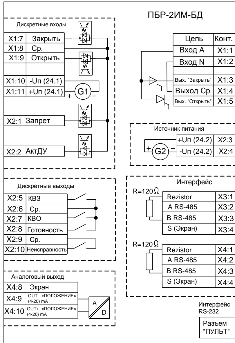
Рисунок Н.4 – Схема ПБР-2ИМ-БД-XX-СУ
