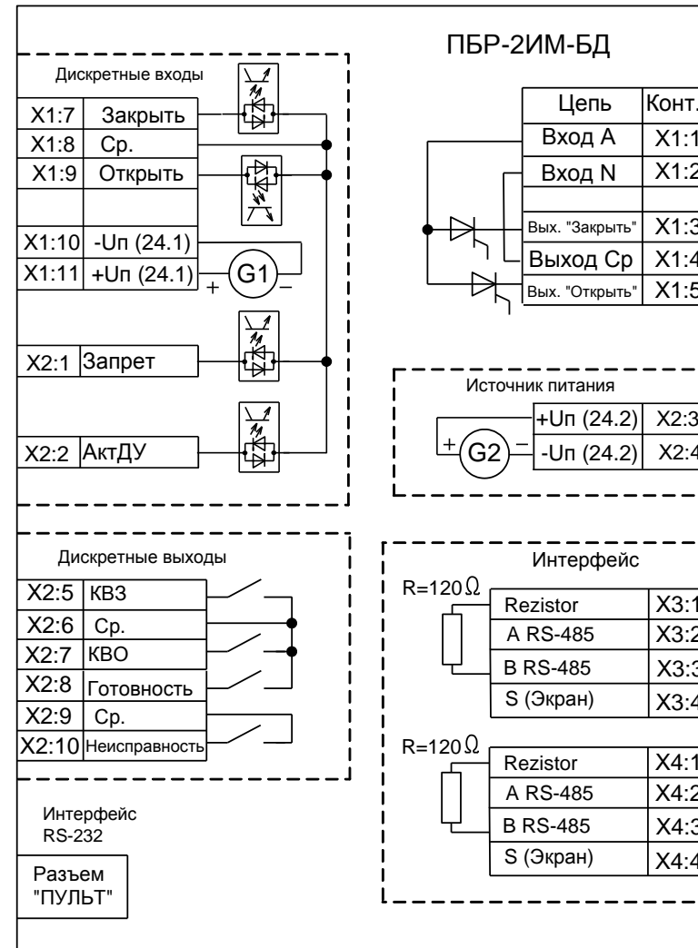
Рисунок Н.2 – Схема ПБР-2ИМ-БД-XX-С
