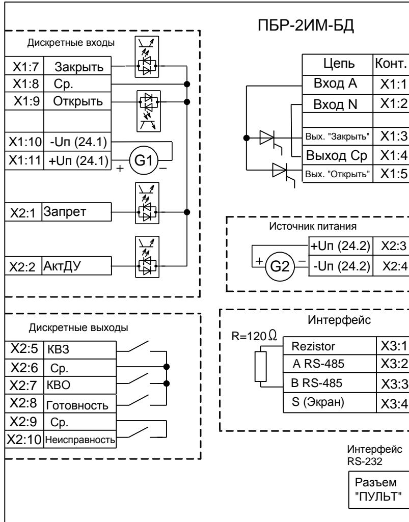
Рисунок Н.1 – Схема ПБР-2ИМ-БД-XX
