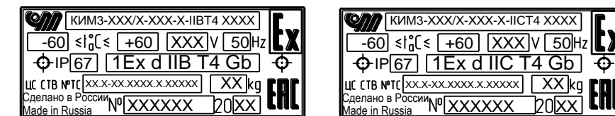
Рисунок Е.2 – Маркировочные таблички
