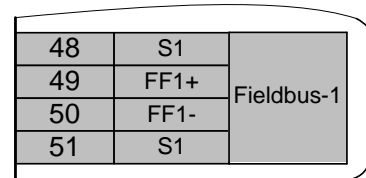
в) контроллеры с опцией "Fieldbus-1", остальное см. рисунок И.5а
