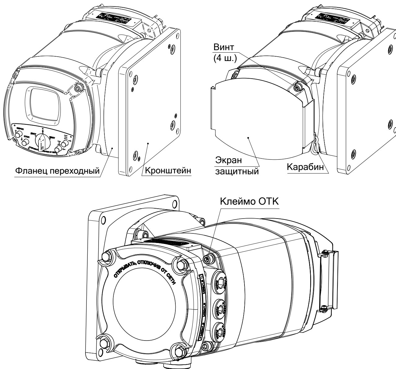
Рисунок 1 – Внешний вид контроллера
