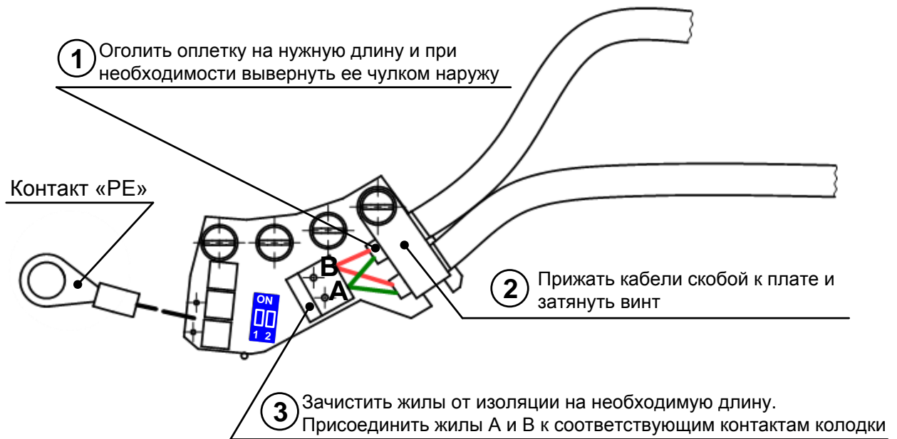
Рисунок Р.2 – Подключение цепей Profibus DP для канала 1
