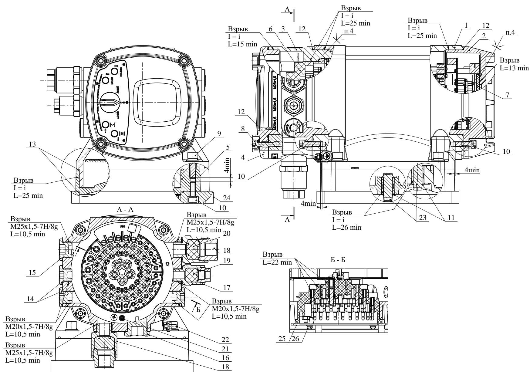
Рисунок Е.1 – Контроллер КИМ3
