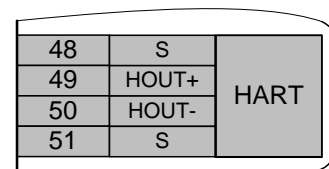
г) контроллеры с опцией "HART", остальное см. рисунок И.5а
