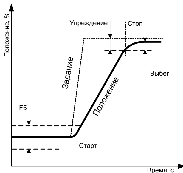
Рисунок 11 – Алгоритм работы позиционера
