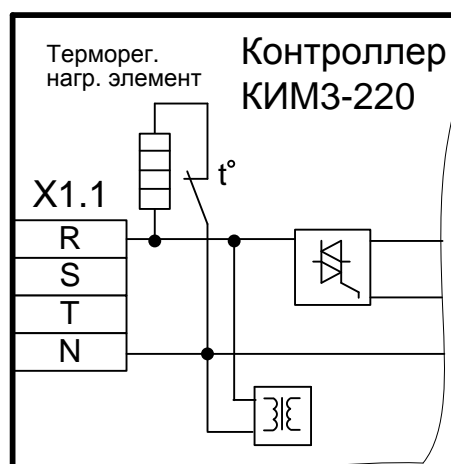
Рисунок И.7 – Схема контроллера КИМ3-220 (остальное см. рисунки И.1-И.6)
