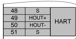
б) контроллеры с опцией "HART", остальное см. рисунок И.6а
