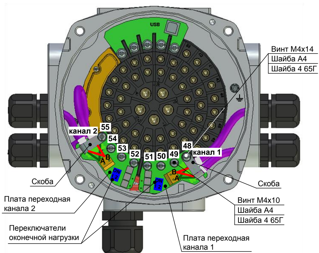
Рисунок Р.1 – Установка плат переходных
