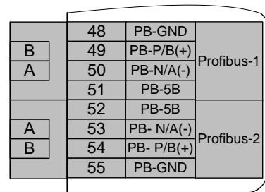
б) контроллеры с опциями "Profibus-1", "Profibus-2", остальное см. рисунок И.5а
