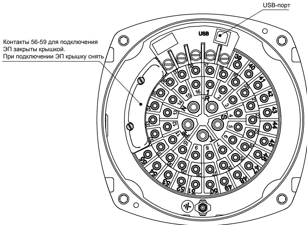
Рисунок К.1 – Клеммная колодка контроллера
